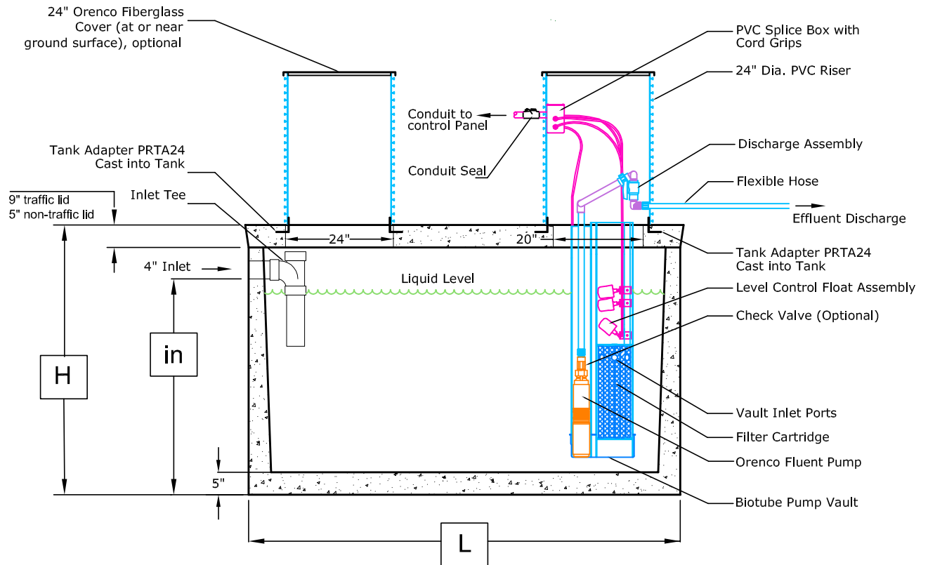
LONGITUDINAL SECTION
