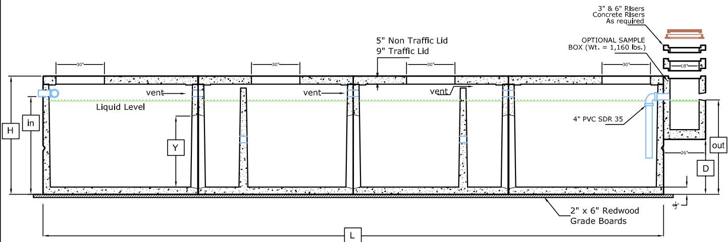
LONGITUDINAL SECTION
