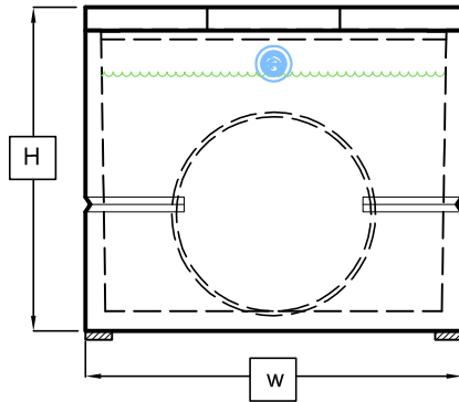
END ELEVATION
