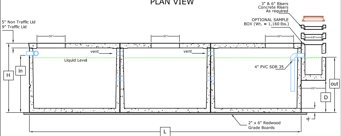
LONGITUDINAL SECTION
