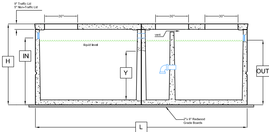
LONGITUDINAL SECTION
