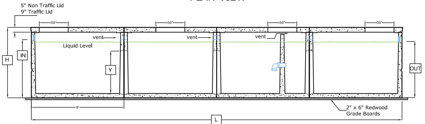
LONGITUDINAL SECTION
