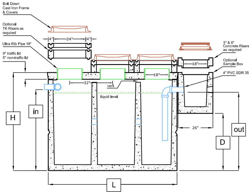
LONGITUDINAL SECTION
