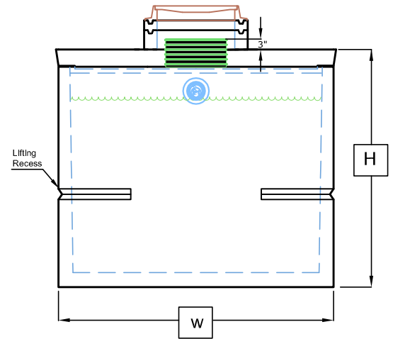
END ELEVATION
