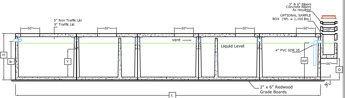
LONGITUDINAL SECTION
