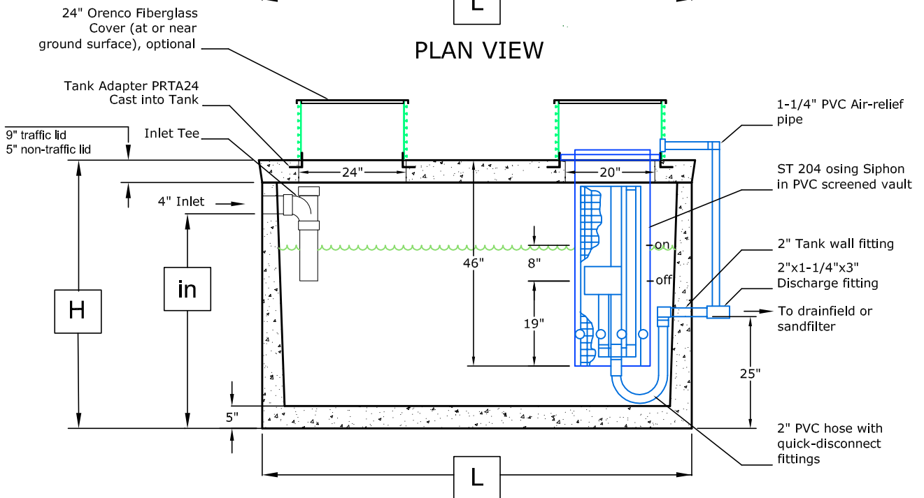
LONGITUDINAL SECTION
