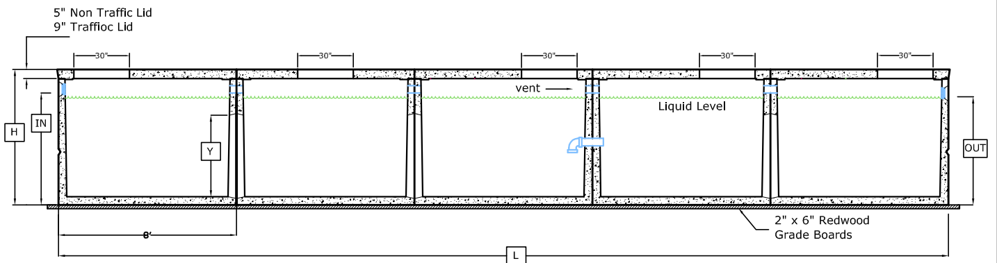
LONGITUDINAL SECTION
