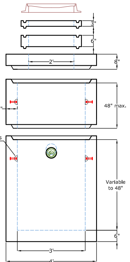
END ELEVATION
