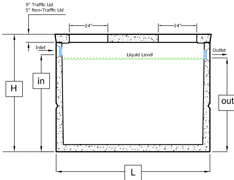
LONGITUDINAL SECTION
