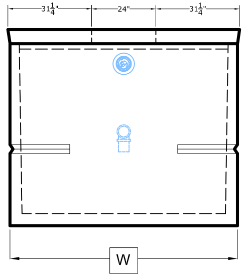
END ELEVATION
