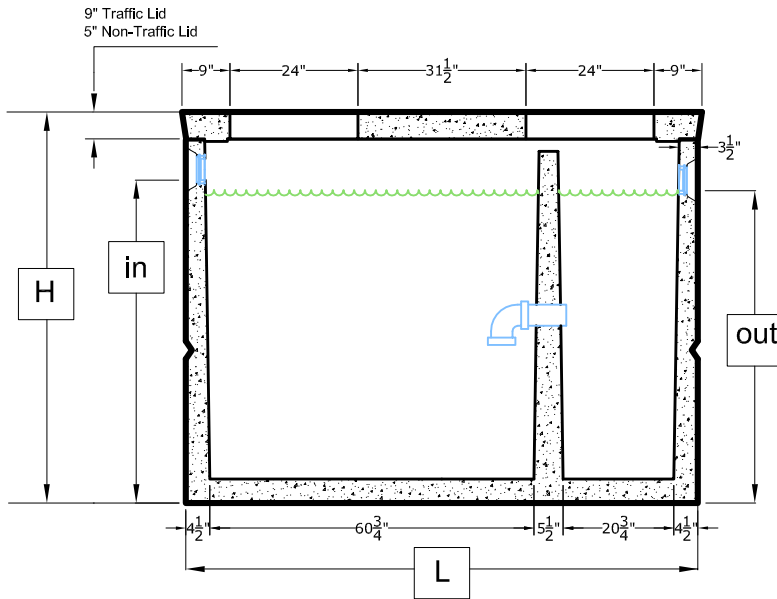
LONGITUDINAL SECTION
